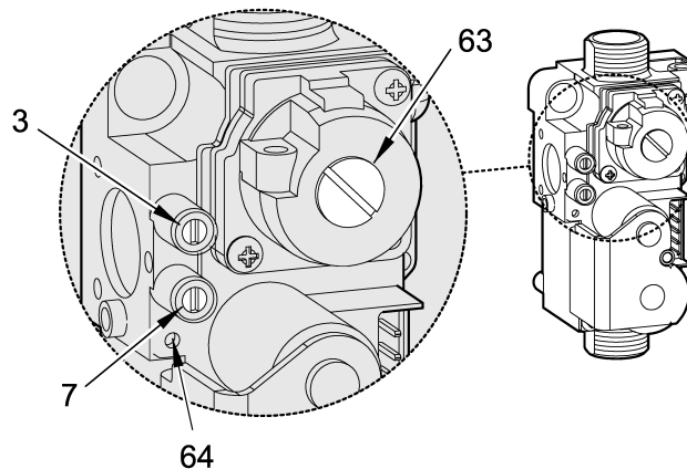
21 pav. Dujų armatūra.
