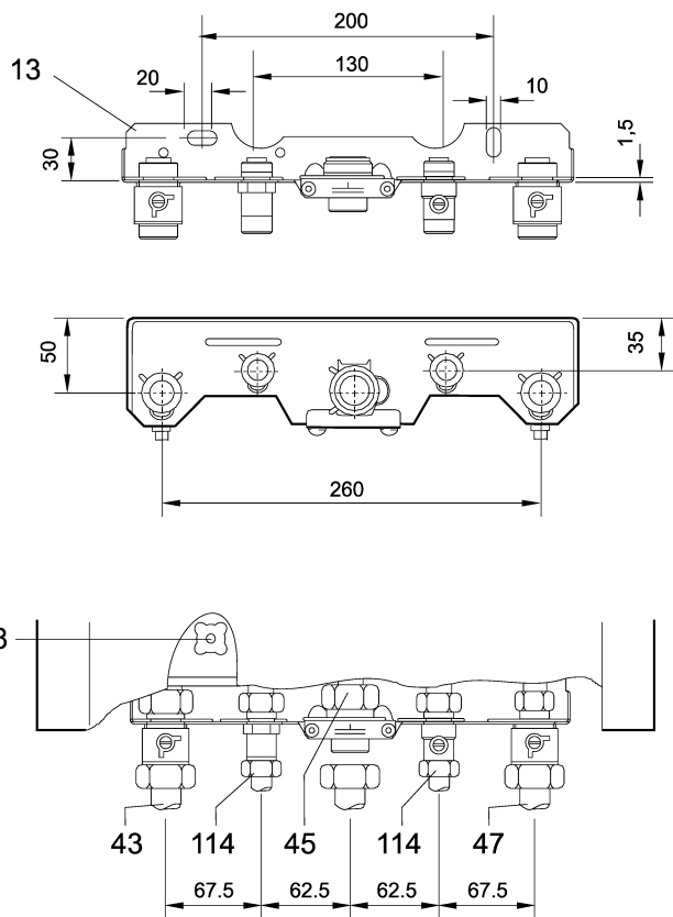
7 pav. Montažinė plokštė
