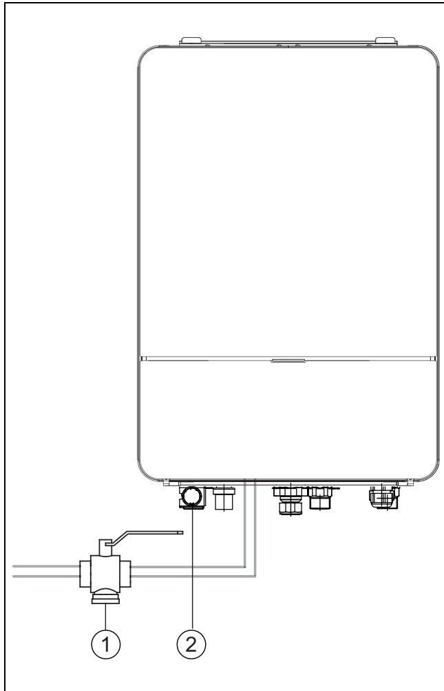
Pav. 7 Vidinis blokas AWB
