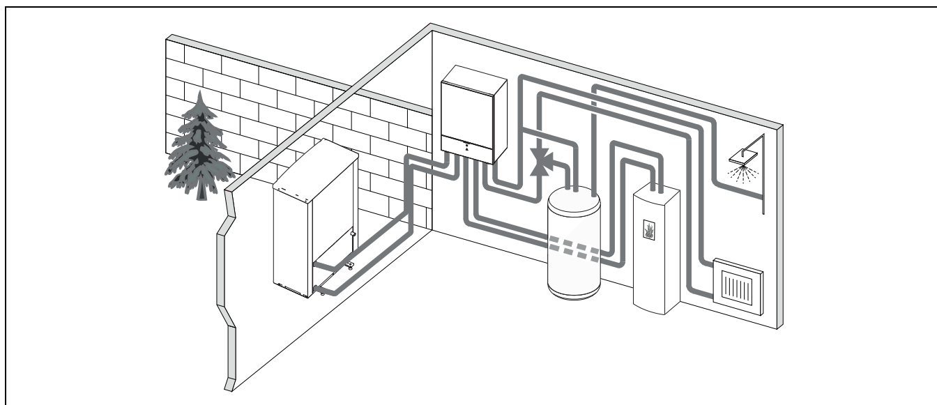
Pav. 3 Šilumos siurblys Compress 7000i AW, vidinis blokas AWB be elektrinio kaitintuvo, išorinė karšto vandens talpykla ir išorinis papildomas kaitintuvas
