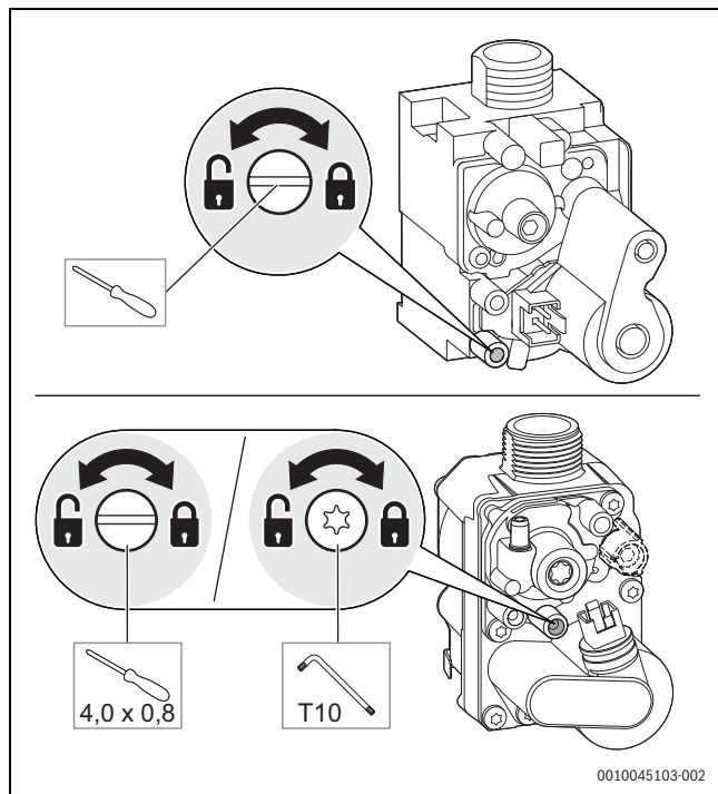
Pav. 46 Dujų prijungimo slėgio matavimas
