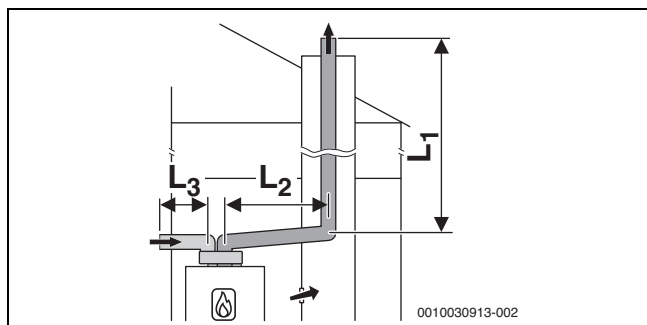
Pav. 12 Standi išmetamųjų dujų sistema pagal C 53 šachtoje ir oro-išmetamųjų dujų kanalas su atskirais vamzdžiais oro tiekimui ir išmetamųjų dujų išvedimui pastatymo patalpoje
