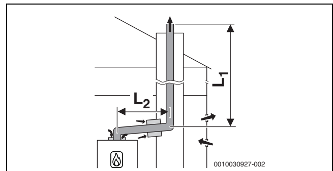
Pav. 17 Standus dujų išvedimo kanalas šachtoje pagal B 23p /B 53p su nuo patalpos oro priklausančia oro tiekimo linija ant įrenginio ir koncentrinu jungiamuoju elementu tarp pastatymo patalpos ir šachtos
