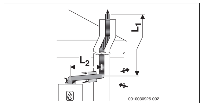
Pav. 18 Lankstus dujų išvedimo kanalas šachtoje pagal B 23p /B 53p su nuo patalpos oro priklausančia oro tiekimo linija ant įrenginio ir koncentrinu jungiamuoju elementu tarp pastatymo patalpos ir šachtos
