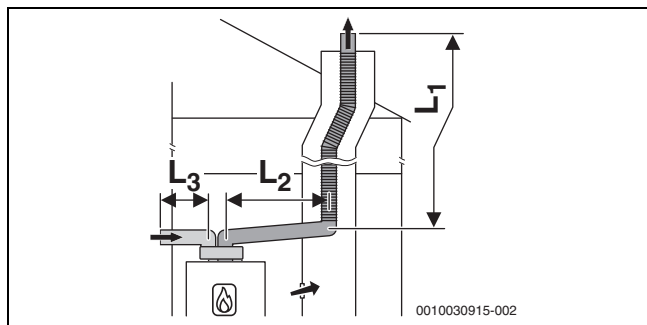
Pav. 13 Lanksti išmetamųjų dujų sistema pagal C 53 šachtoje ir oro-išmetamųjų dujų kanalas su atskirais vamzdžiais oro tiekimui ir išmetamųjų dujų išvedimui pastatymo patalpoje
