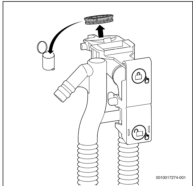
Pav. 66 Sandarinimo detalės kondensato sifono viršuje nuėmimas
