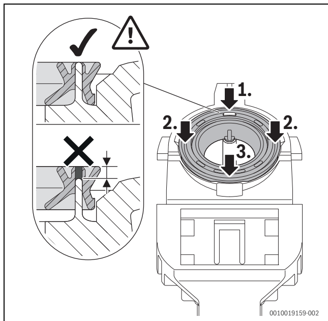
Pav. 68 Sandarinimo detalės prispaudimas
