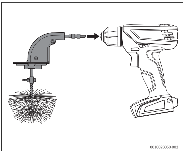
Pav. 60 Šepetio sujungimas su akumuliatoriniu suktuvu
