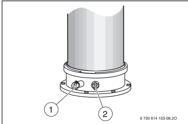
Pav. 50 Išmetamųjų dujų atvamzdžiai ir degimui naudojamo oro matavimo atvamzdžiai
