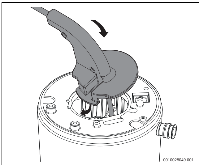
Pav. 59 Šepetio įstatymas į šiluminį bloką
