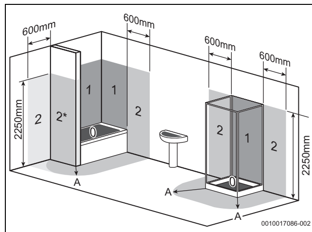
Pav. 22 Apsaugos zonos (ilustracijos pavyzdys)
