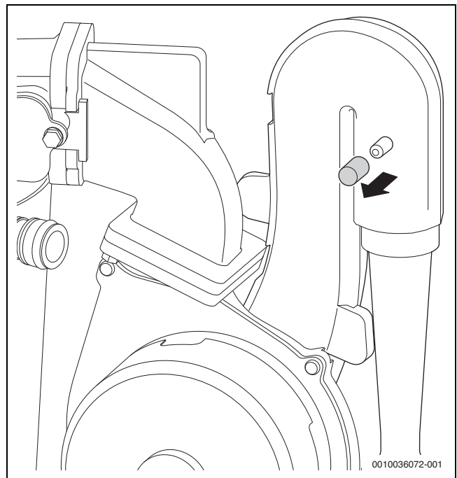
Pav. 51 Matavimo atvamzdis ant maišymo įrenginio
