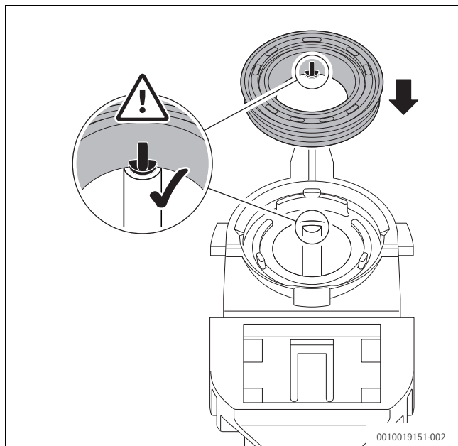
Pav. 67 Naujos sandarinimo detalės ant kondensato sifono uždėjimas
