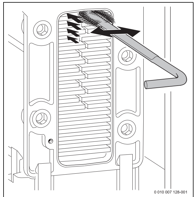
Pav. 50 Šiluminio bloko valymas šepečiu
