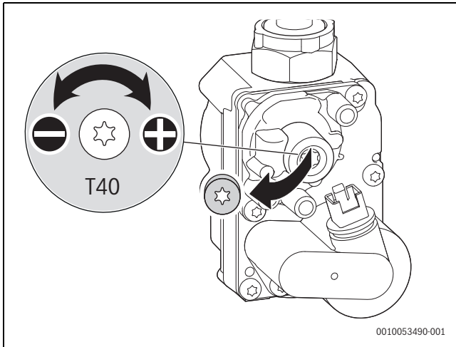
Pav. 40 Nustatykite CO 2 arba O 2 kiekį
