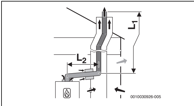
Pav. 17 Lanksti dujų išvedimo linija šachtoje pagal B 53p su nuo patalpos oro priklausančia oro tiekimo linija ant įrenginio ir vienos sienelės išmetamųjų dujų kanalu patalpoje, kurioje statomas įrenginys; galinės ventiliacijos anga šachtoje
