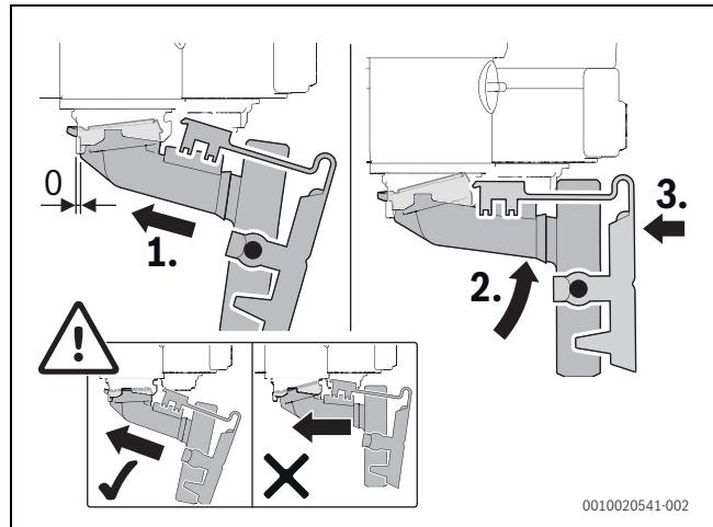
Pav. 53 Kondensatsiphon
