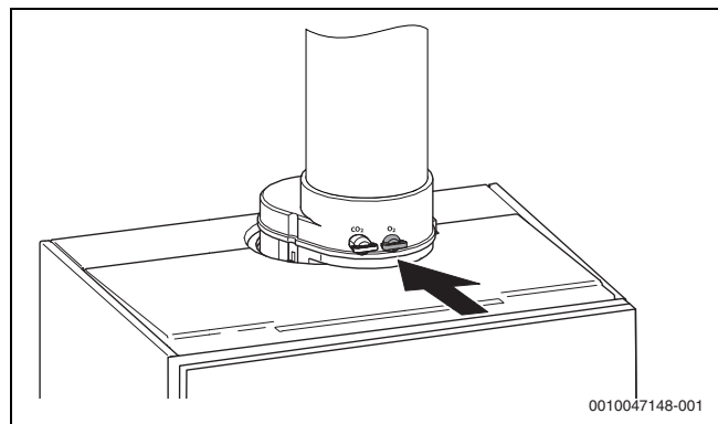
Pav. 39 Išmetamųjų dujų matavimo jungtis
