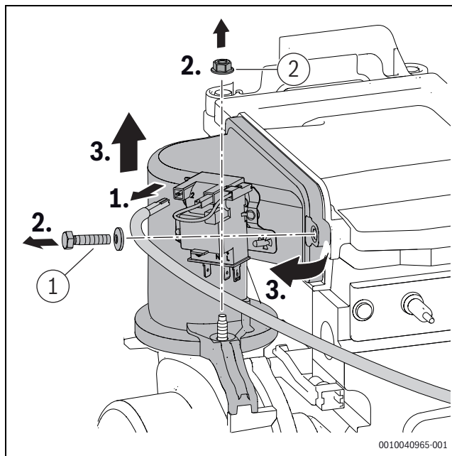
Pav. 46 Maišymo įrenginio išmontavimas
