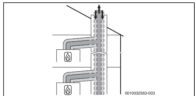
Pav. 18 Būdas, kai prie dūmtraukio jungiami keli įrenginiai pagal C (10)3x su koncentrinio oro-išmetamųjų dujų kanalu pastatymo patalpoje
