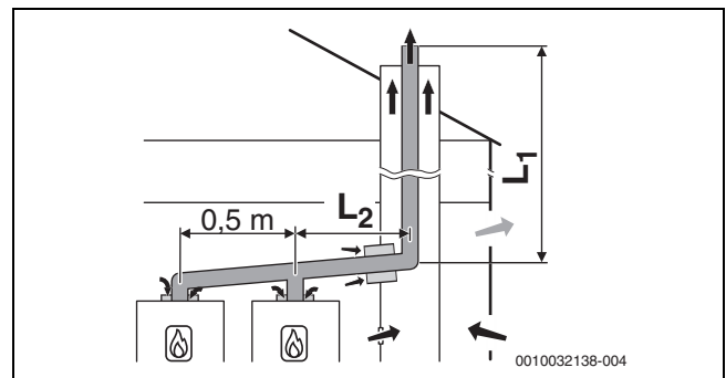
Pav. 22 Kaskada su 2 įrenginiais: standi išmetamųjų dujų sistema šachtoje pagal B 53p su nuo patalpos oro priklausančia oro tiekimo linija ant įrenginio ir vienos sienelės išmetamųjų dujų kanalu patalpoje, kurioje statomas įrenginys, galinės dalies ventiliacijos anga šachtoje
