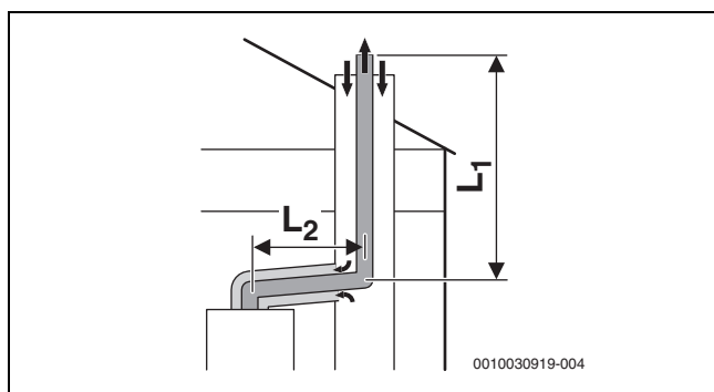
Pav. 14 Standi išmetamųjų dujų sistema pagal C 93x šachtoje ir koncentrinis jungiamasis laidas patalpoje, kurioje statomas įrenginys
