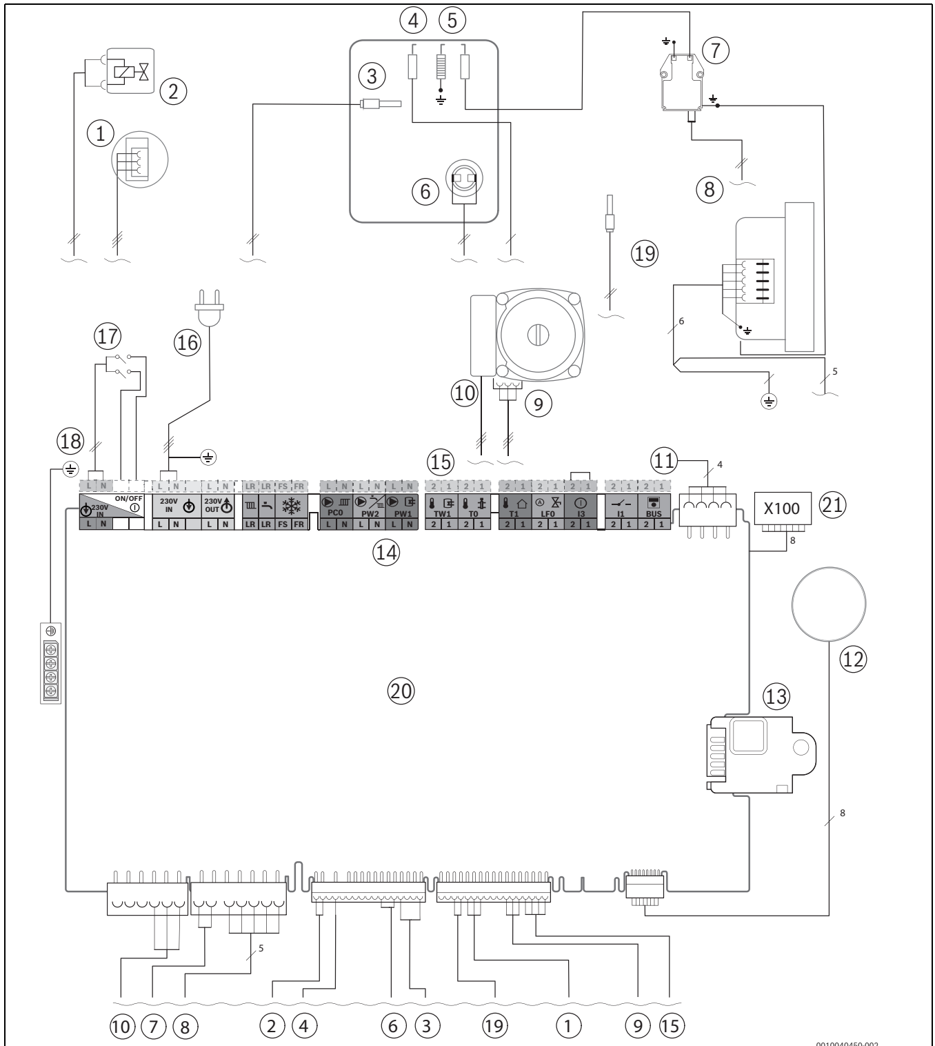
Pav. 59 Elektros laidų montavimas
